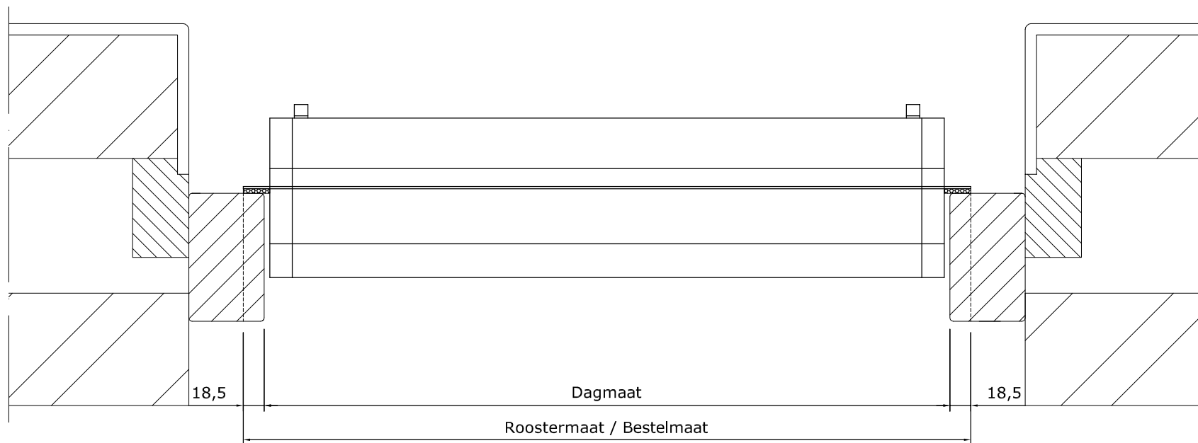
Duco Ventilation & Sun Control - FireMax 'ZR' - Compacte halfplaatsing (verlengde buitenkap)
