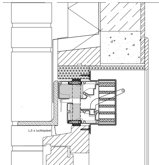
Duco Ventilation & Sun Control - FireMax 'ZR' - Compacte halfplaatsing (onzichtbare plaatsing)
