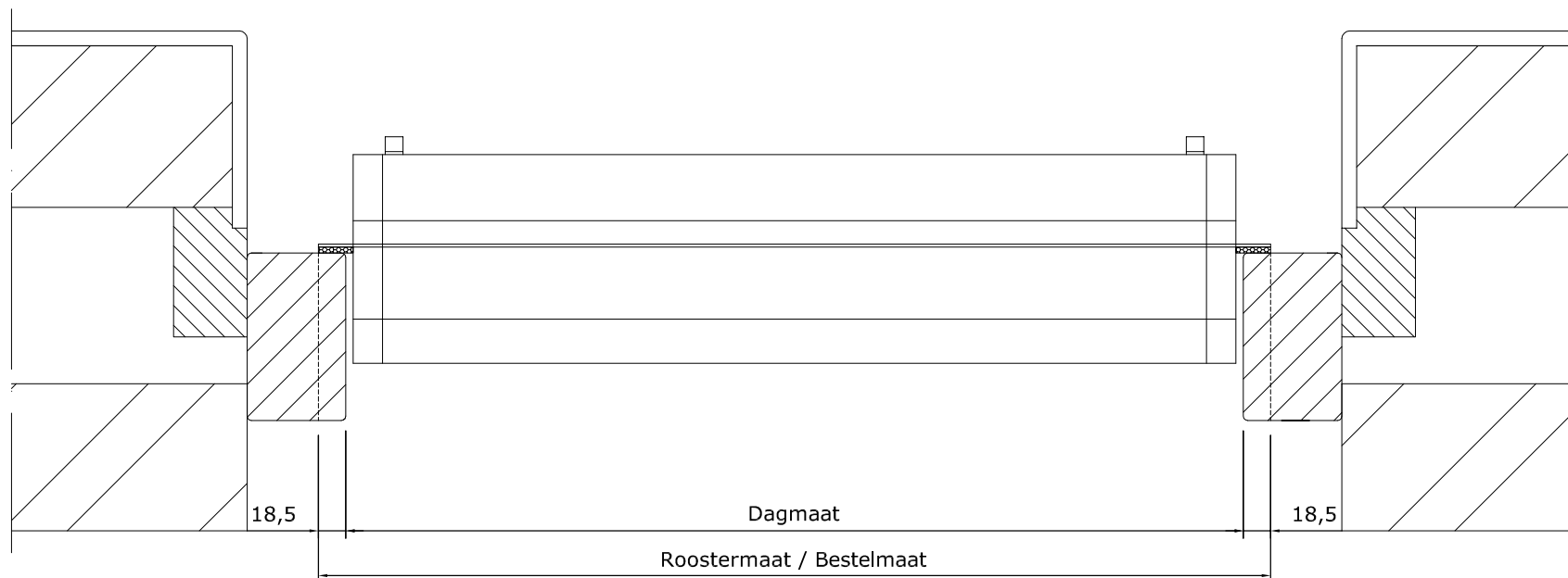
Duco Ventilation & Sun Control - FireMax 'ZR' - Compacte halfplaatsing (onzichtbare plaatsing)
