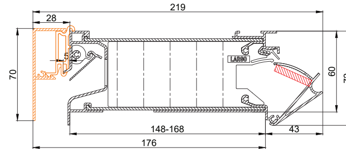
DucoTop 60 ZR Largo
