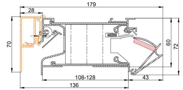
DucoTop 60 ZR Medio
