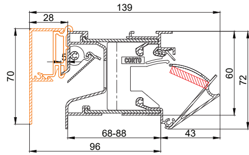
DucoTop 60 ZR Corto
