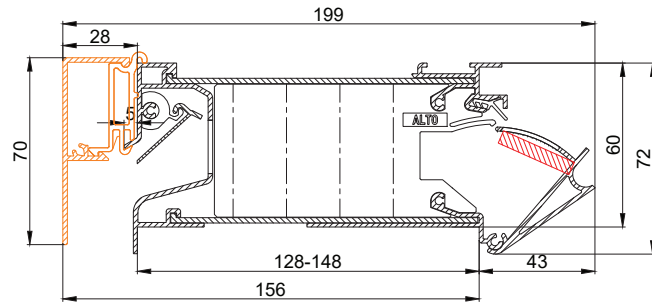
DucoTop 60 ZR Alto
