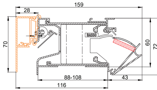
DucoTop 60 ZR Basso
